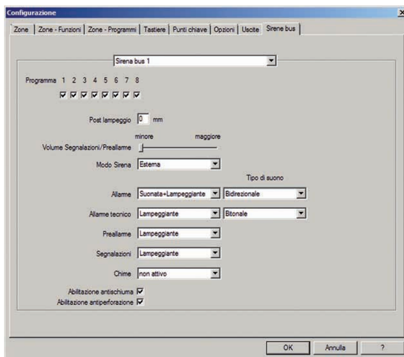
Videata programmazione sirena Bus da PC
